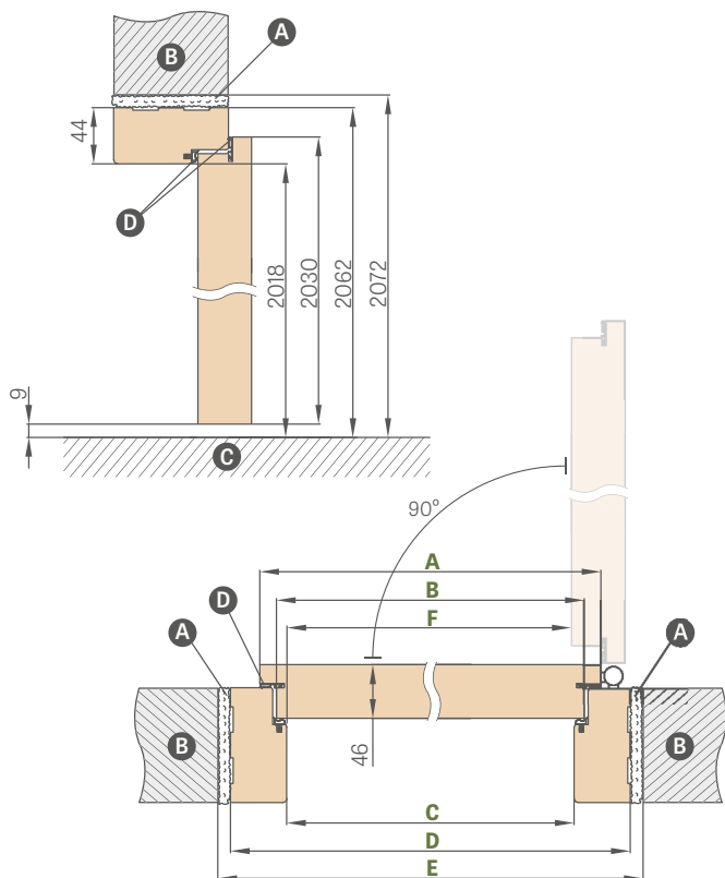
ŠEMA FIKSNOG DOVRATNIKA HERSE SET
