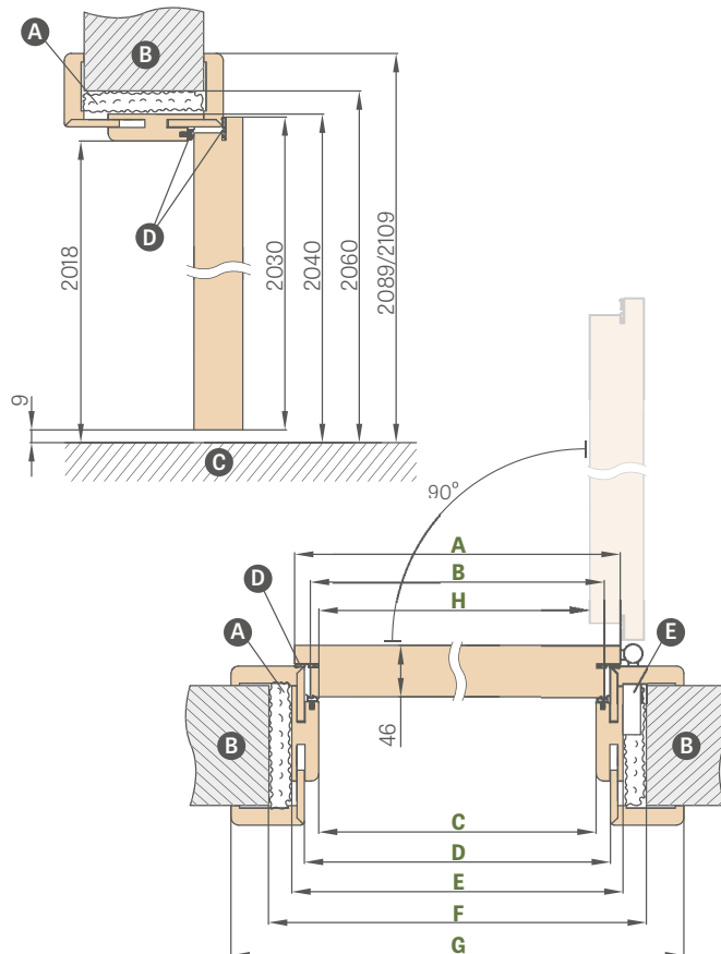
ŠEMA PODESIVOG DOVRATNIKA HERSE SET
