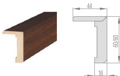
STANDARDNI KUTNIK ZA PODESIVI DOVRATNIK
