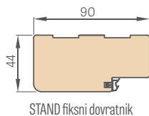
STAND fiksni dovratnik
