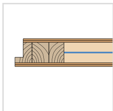
KRILO 46 mm ojačano čeličnim limom
