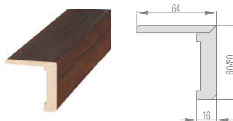
KUTNIK S PRODULJENIM PEROM ZA PODESIVI DOVRATNIK
